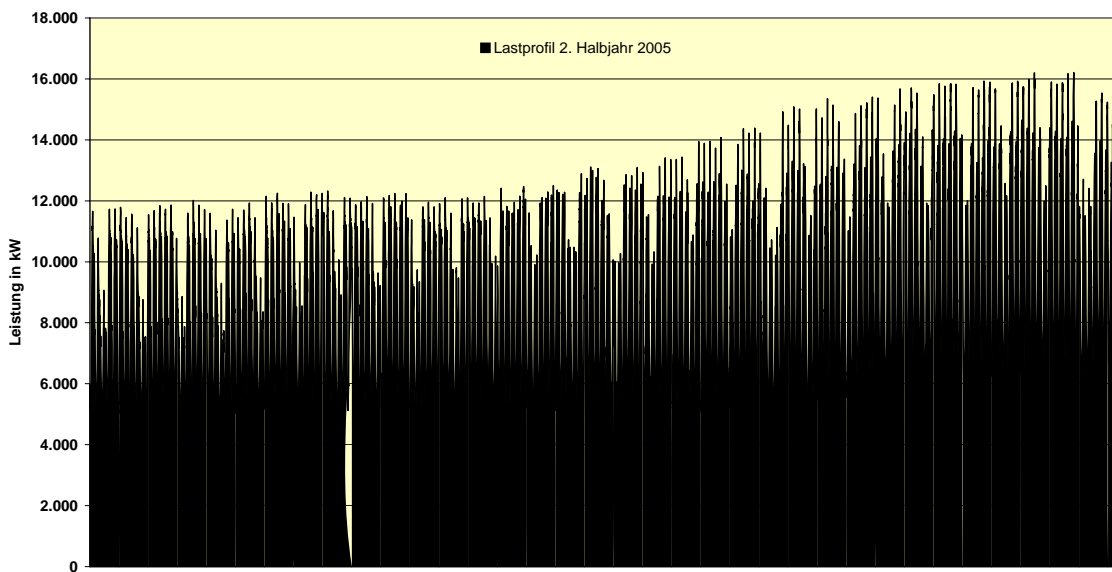
Lastprofil Strom 2. Halbjahr 2005 Netzgebiet Schwedt
