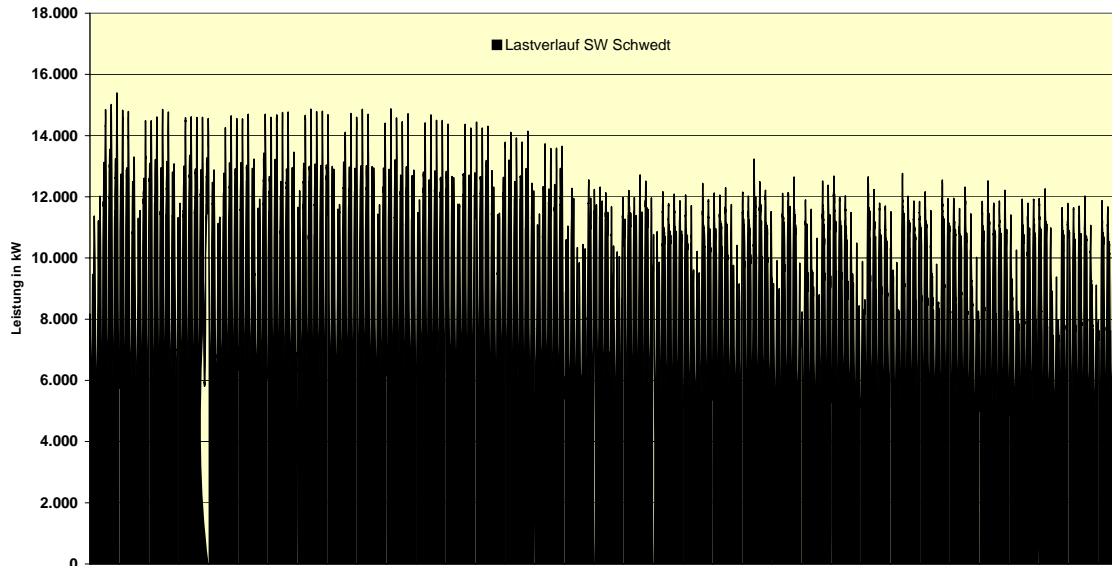
Lastprofil Strom 1. Halbjahr 2005 Netzgebiet Schwedt
