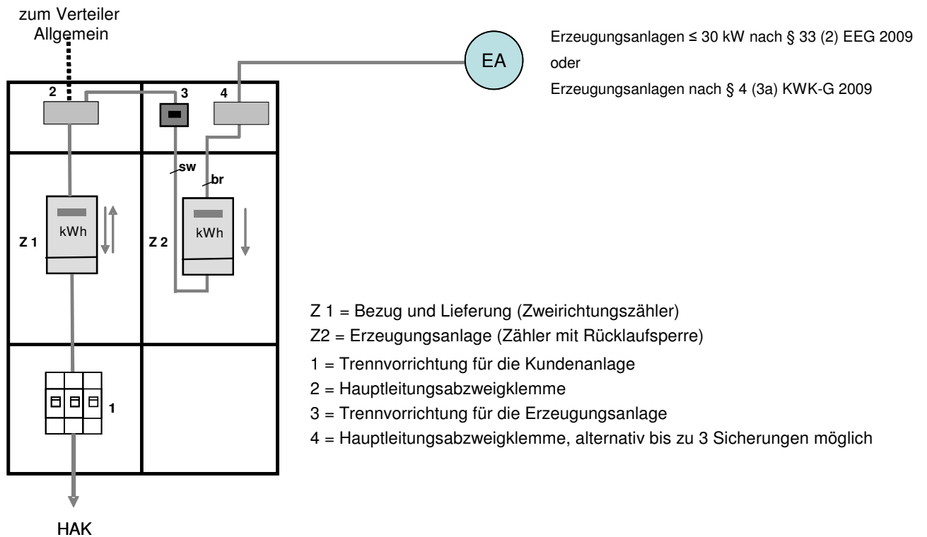
Abbildung 2: Anschlussvariante bei zentralem konventionellem Zählerplatz mit Drei-Punkt-Befestigung
