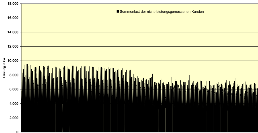
Summenlast der nicht-leistungsgemessenen Kunden 1. Halbjahr 2005 Netzgebiet Schwedt
