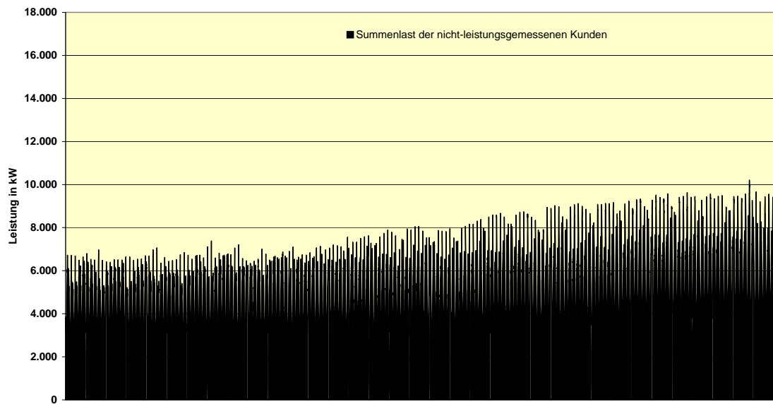
Summenlast der nicht-leistungsgemessenen Kunden 2. Halbjahr 2005 Netzgebiet Schwedt
