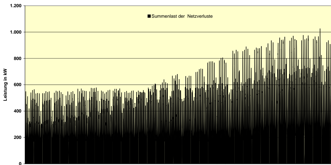
Summenlast der Netzverluste Strom 2. Halbjahr 2005 Netzgebiet Schwedt
