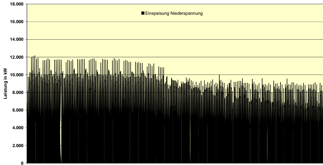
Stromeinspeisungen in Niederspannung 1. Halbjahr 2005 Netzgebiet Schwedt
