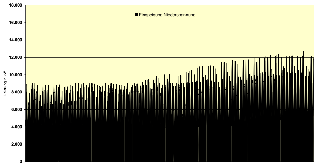
Stromeinspeisungen in Niederspannung 2. Halbjahr 2005 Netzgebiet Schwedt
