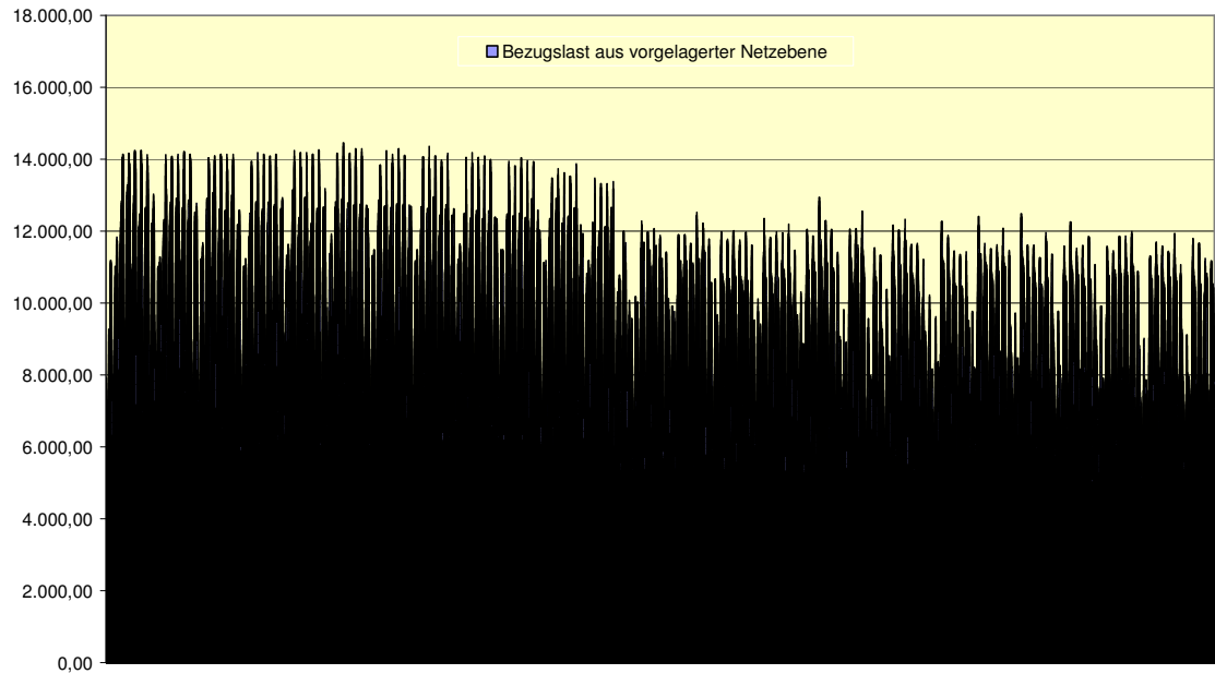
Bezugslast aus vorgelagerter Netzebene 1. Halbjahr 2005 Netzgebiet Schwedt
