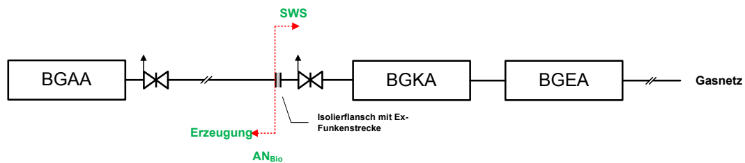
Abb. 2 Schemaskizzen Rechtsträgerschafts-/Eigentumsgrenzen Biogaseinspeisung zwischen Anschlussnehmer und Netzbetreiber
