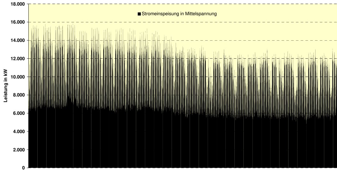
Stromeinspeisung in Mittelspannung 1. Halbjahr 2006 Netzgebiet Schwedt
