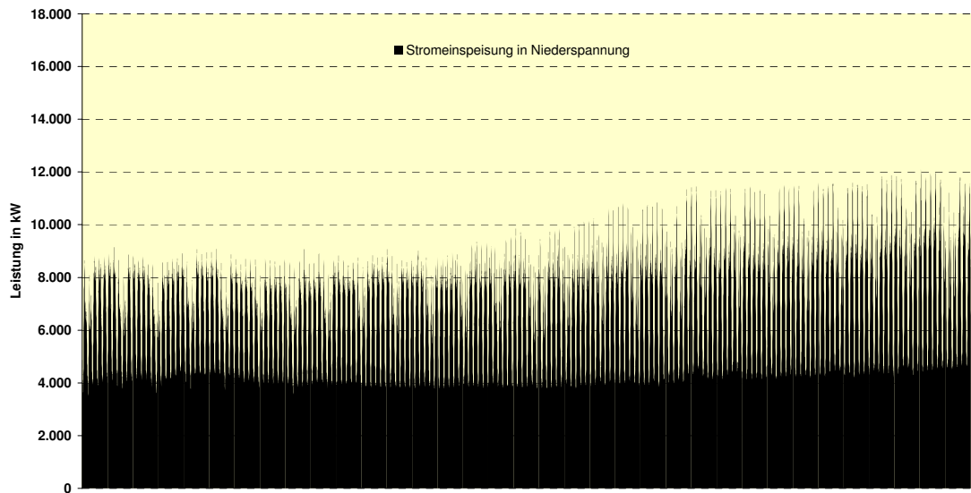
Stromeinspeisung in Niederspannung 2. Halbjahr 2006 Netzgebiet Schwedt
