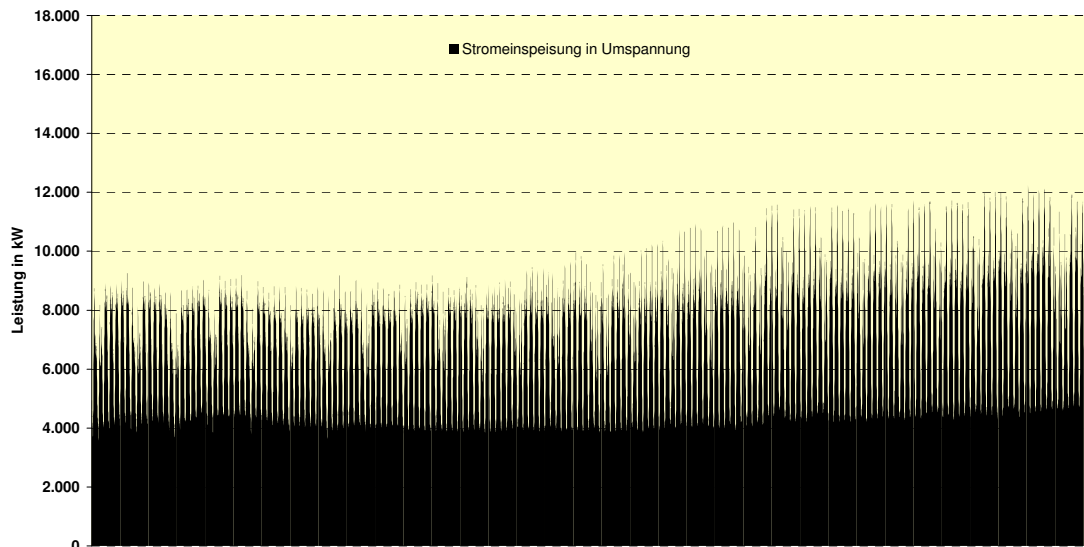
Stromeinspeisung in Umspannung 2. Halbjahr 2006 Netzgebiet Schwedt
